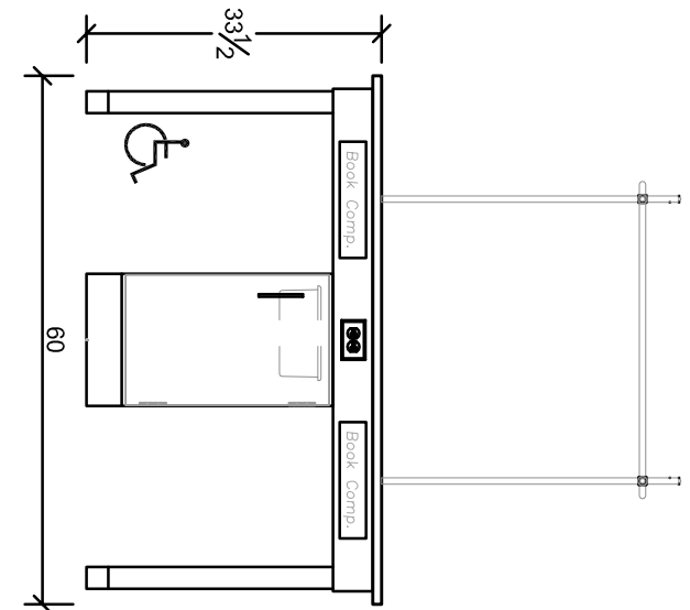
ELEVATION 15B
